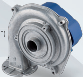
NG40-E M28 (divergent venturi "28")
